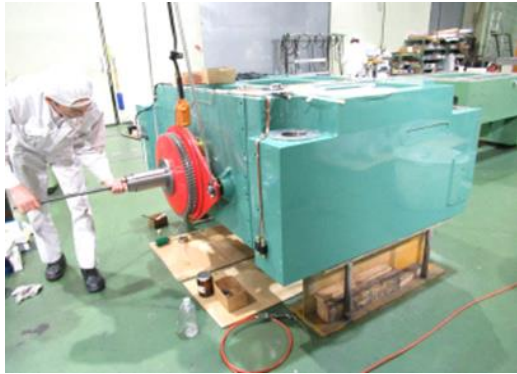
⑤ ユニット組み (シャフト挿入作業)
